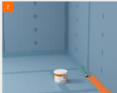
2 fermacell™ vloeibare folie in de hoeken aanbrengen
