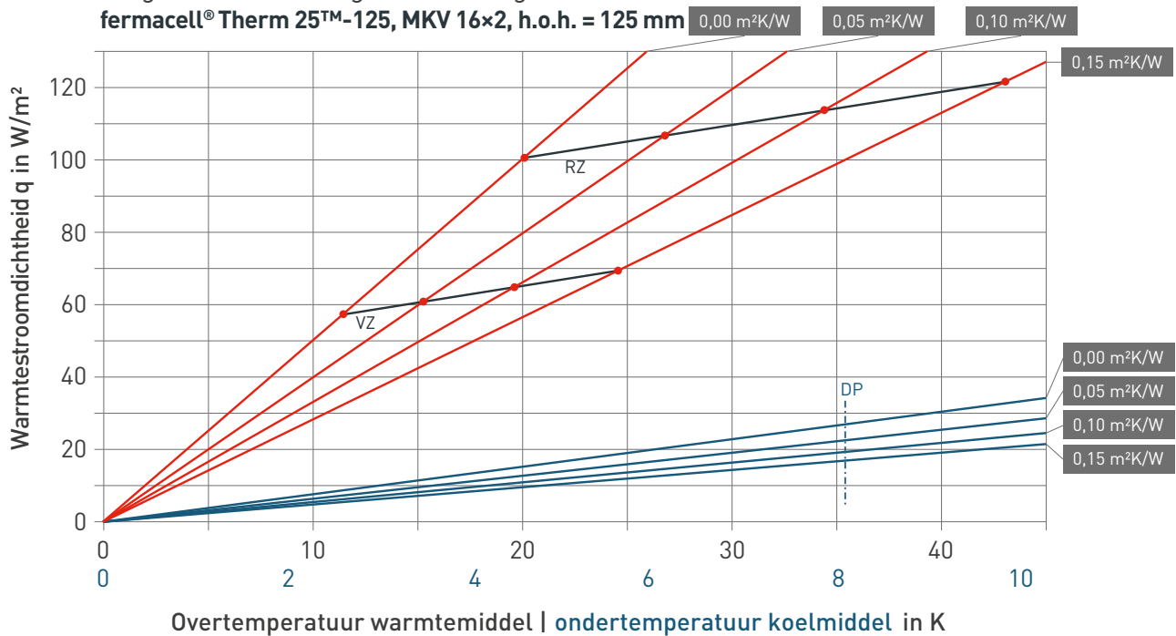
Diagram verwarmings- en koelingskenmerken
