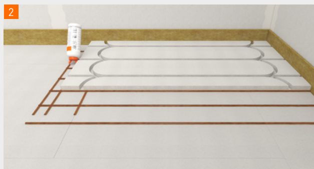
De lijmrillen voor de voegverlijming van het fermacell® Therm25™ element aanbrengen.
