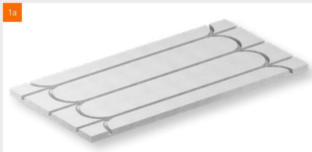
fermacell® Therm25™ Vloerverwarmingselement met leidingsleuven met sleufafstand 167 mm voor de montage van 16mm verwarmingsleidingen, toepassing in het grotere oppervlak.
