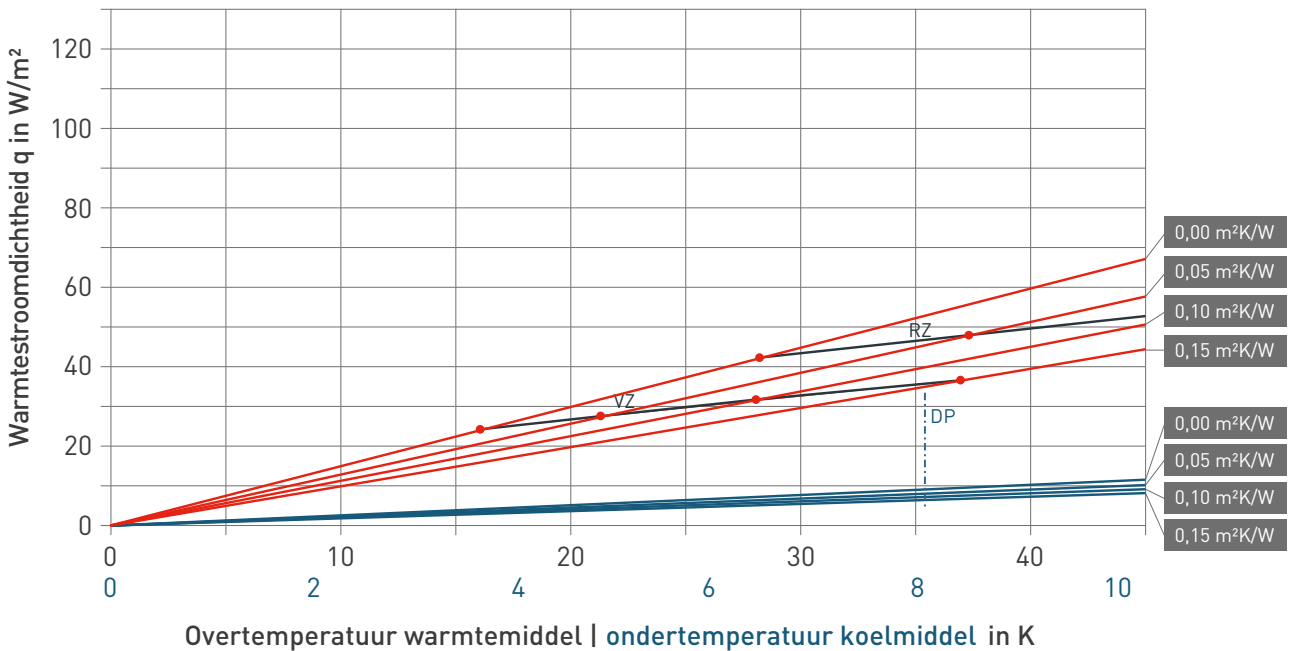
Diagram verwarmings- en koelingskenmerken fermacell® Therm25™-10, MKV 16 × 2, h.o.h. = 334 mm
