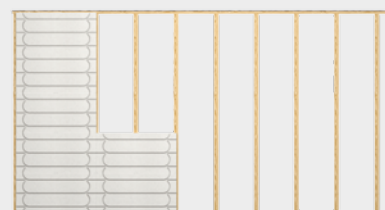
Montage van fermacell® Therm25™ vloerverwarmings-elementen op de achterconstructie (schroeven 40 mm of nieten 50 mm)
