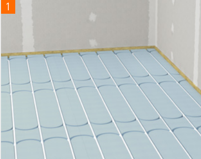
1 De aangebrachte vloerverwarmingsleidingen van 16 mm.
