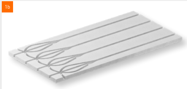
fermacell® Therm25™-125 Vloerverwarmingselement, leidingsleuven met sleufafstand 125 mm voor de montage van 16mm verwarmingsleidingen en betere thermische prestaties, toepassing in het grotere oppervlak.
