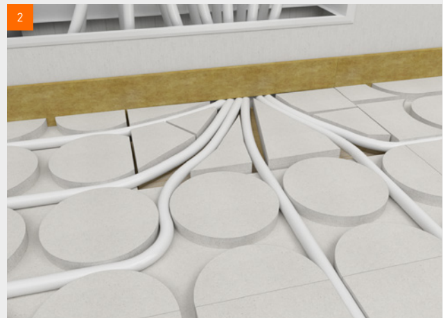
Opvullen met stukken uit fermacell® Therm 25™ of bijvoorbeeld honingraatkorrels.
