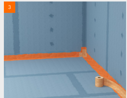
3 De fermacell™ afdichtband in de nog natte vloeibare folie drukken
