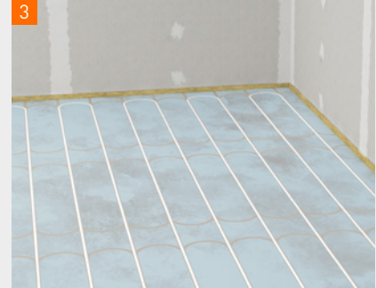
3 fermacell® Therm25™ elementen waarop gipslijm uitgegoten is.
