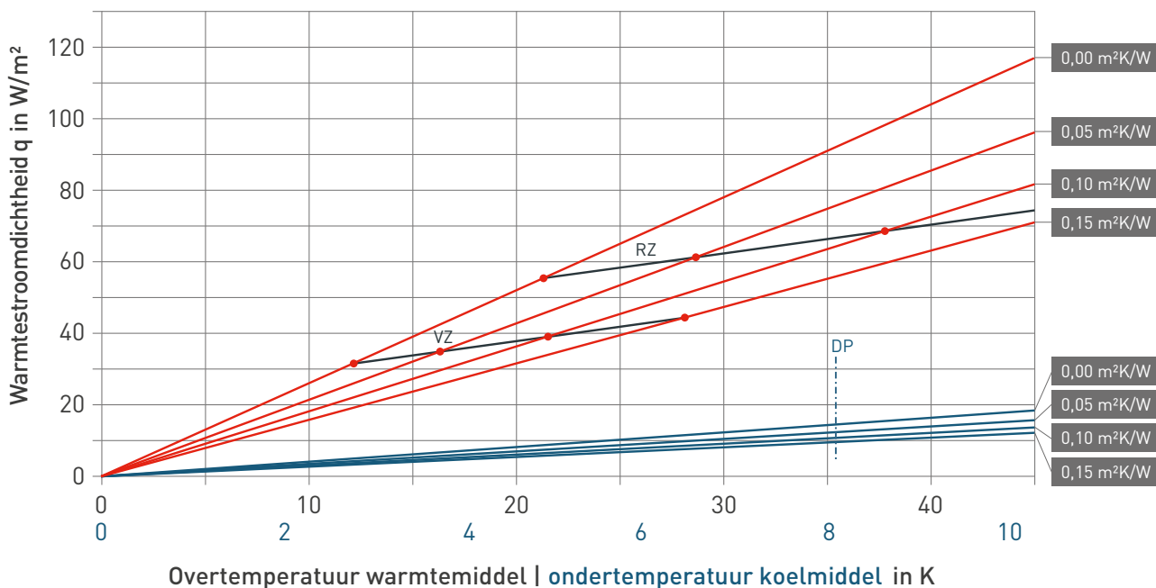
Diagram verwarmings- en koelingskenmerken fermacell® Therm 25™-125, MKV 16x2, h.o.h. = 250 mm
