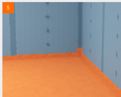
5 De vlakken in W1-l-zones volvlaks aanbrengen
