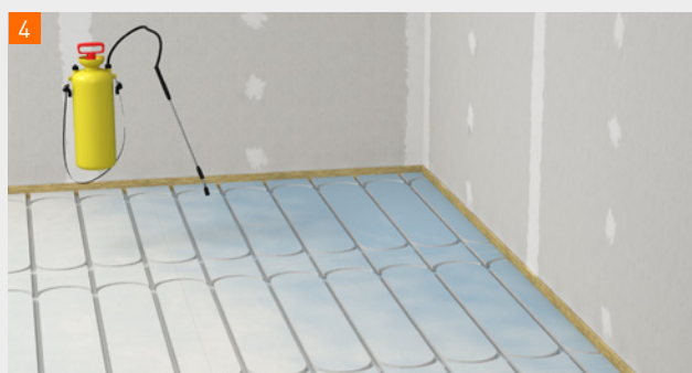
De fermacell® Therm25™ elementen met fermacell™ diepgrond gronderen.
