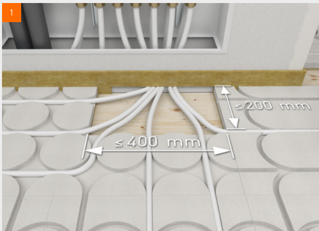
Maximale grootte van de uitsparing 400 x 200 mm voor variant 1.
