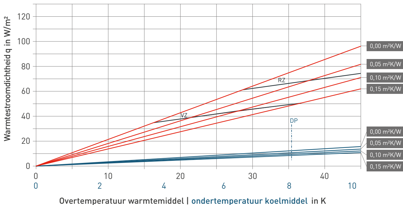
Diagram verwarmings- en koelingskenmerken fermacell® Therm 25™-125, MKV 16x2, h.o.h. = 250 mm
