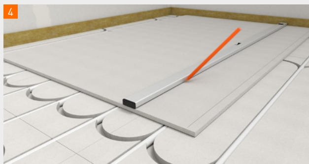
Aftekenen van de bevestigingspunten (raster ong. 167 × 250 mm).
