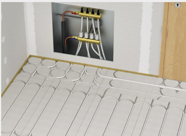
fermacell® Therm25™ element rond ter plaatse van de warmteverdeler met extra ingefreesde sleuven.
