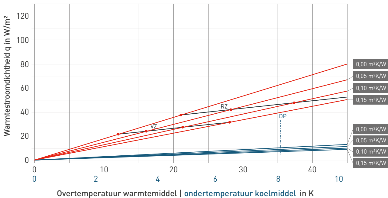
Diagram verwarmings- en koelingskenmerken fermacell® Therm25™-2, MKV 16×2, h.o.h. = 334 mm
