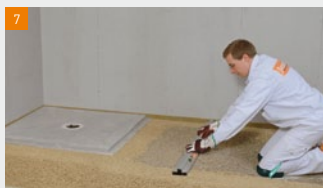
Wanneer het gebonden egalisatiemiddel tussen de dammen gestort is, kan het afreien beginnen
