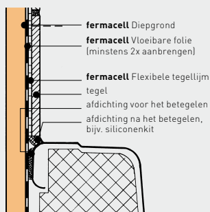
Wandaansluitingen van douchecel of badkuip. Aansluiting aan fermacell montagewand met enkele beplating
